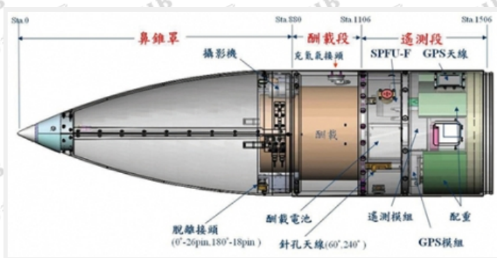
圖 2：探空七號酬載配置圖
