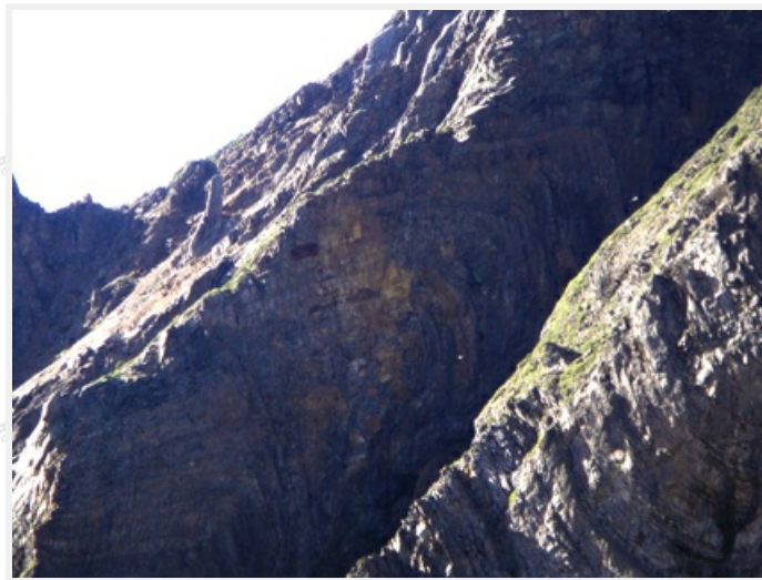
鳳尾岩。位在玉山主峰與東峰之間，北壁有向右上方堆疊的地層紋路， 明顯反映地殼深處的高溫與高壓的擠壓作用
